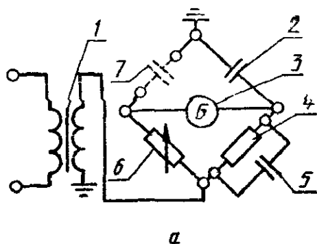
Схема с заземленной диагональю
