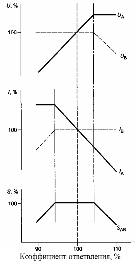
Рисунок 3 — Комбинированное регулирование напряжения (режим v )
