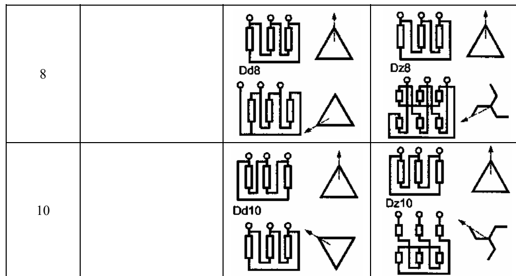
Рисунок Г.2 — Дополнительные схемы и группы соединения обмоток
