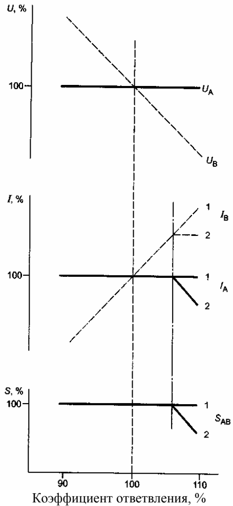
Рисунок 2 — Регулирование напряжения при переменном магнитном потоке (режим b )
