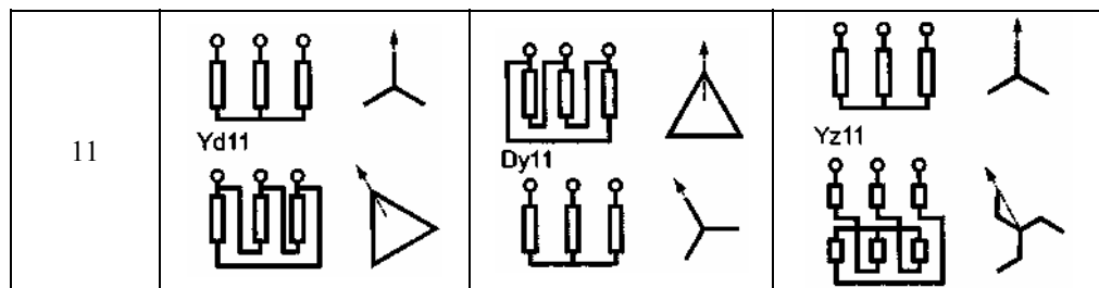
Рисунок Г.1 — Стандартные схемы и группы соединения обмоток
