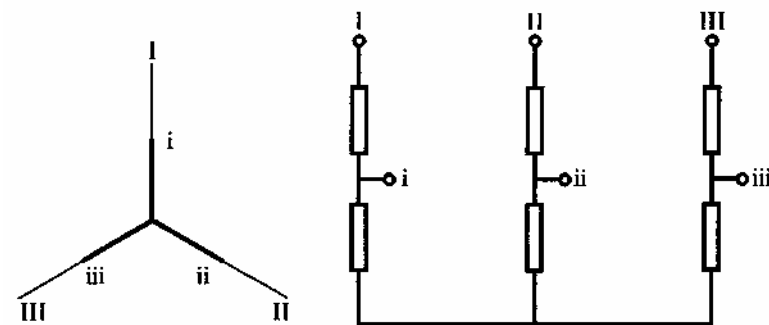
Рисунок Г.3 — Схема и группа соединения обмоток трехфазных автотрансформаторов
